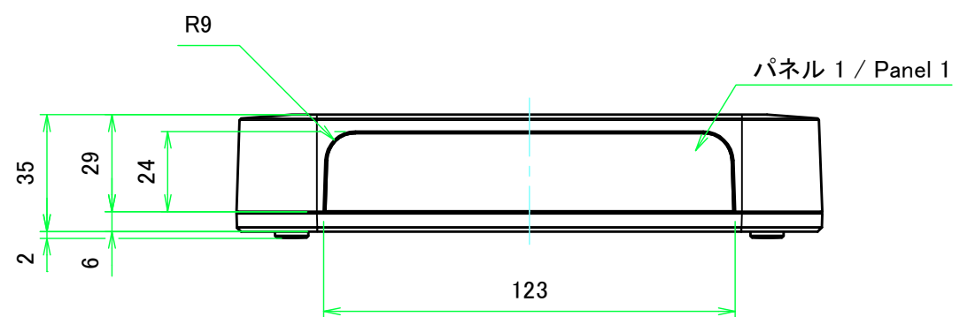
B-B (1:2)
