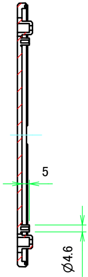
E-E ( 1 : 2.5 )
