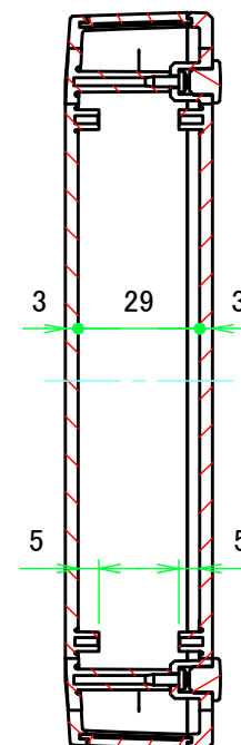
A-A (1:2)
